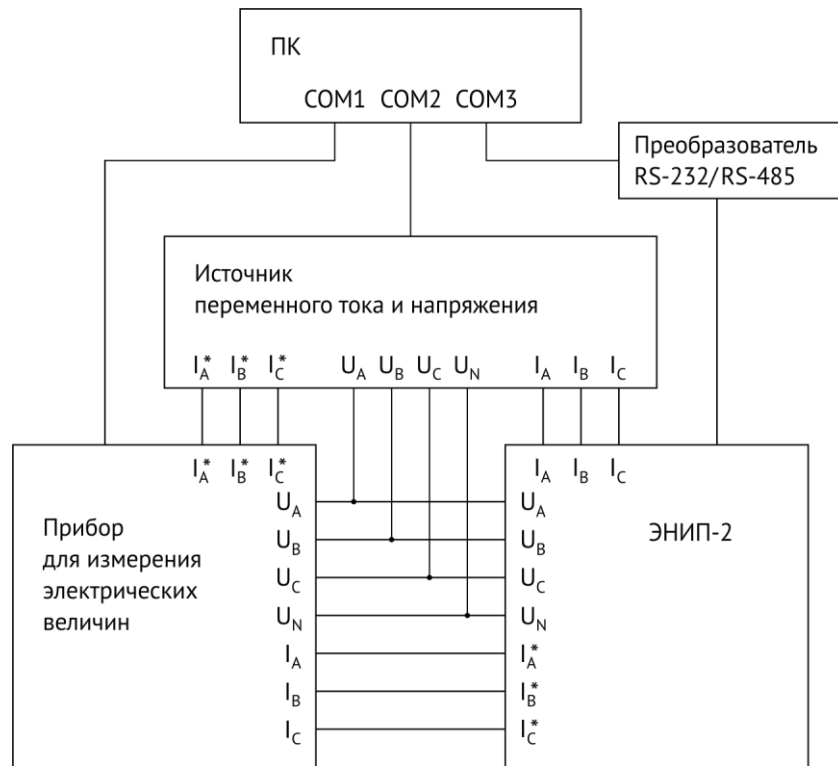
Рисунок 3 – Схема рабочего места при поверке преобразователей ЭНИП-2
